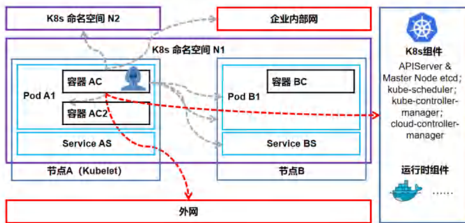
图 7-2 传统或新型的 K8s 攻击利用方式
